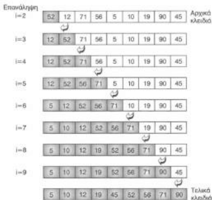
Σχήμα 3.1. Ταξινόμηση ευθείας εισαγωγής.
