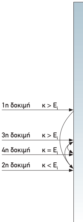
Σχ. 4.2. Δυαδική αναζήτηση
